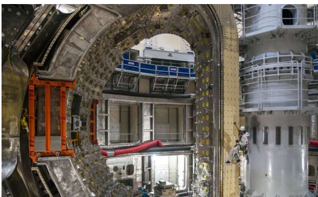
Eine der gewaltigen supraleitenden Magnetspulen, die bei ITER das Fusions-Plasma in der Vakuumkammer einschließen sollen. :Bild: ITER
