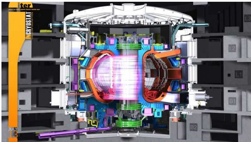
Illustration Fusionsreaktor Iter :Bild: ITER
